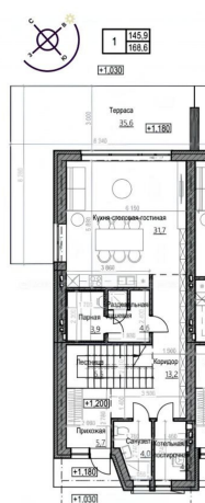
ПЛАН 1 ЭТАЖА
